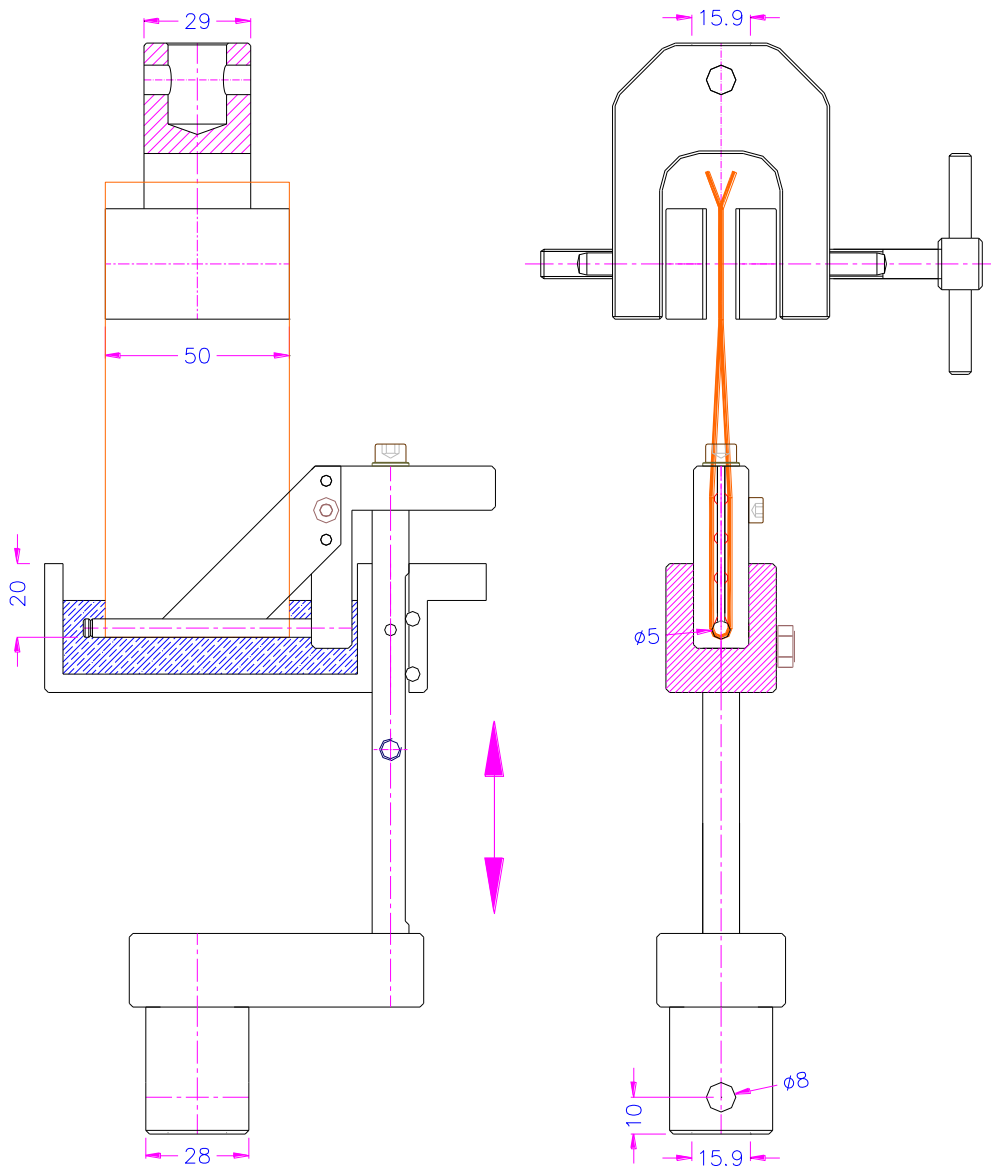
TH240k Kleiner Schraubspannkopf
